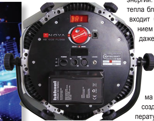
Задняя панель прибора ANOVA – хорошо видны аккумулятор, разъемы, органы управления и дисплей
