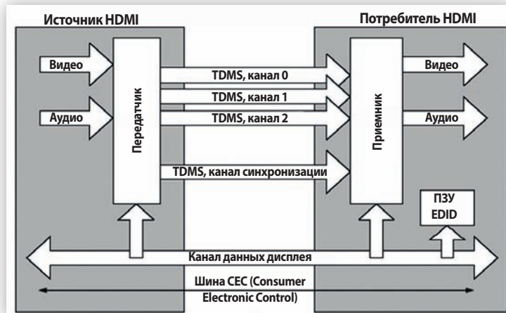
Структурная схема интерфейса HDMI
