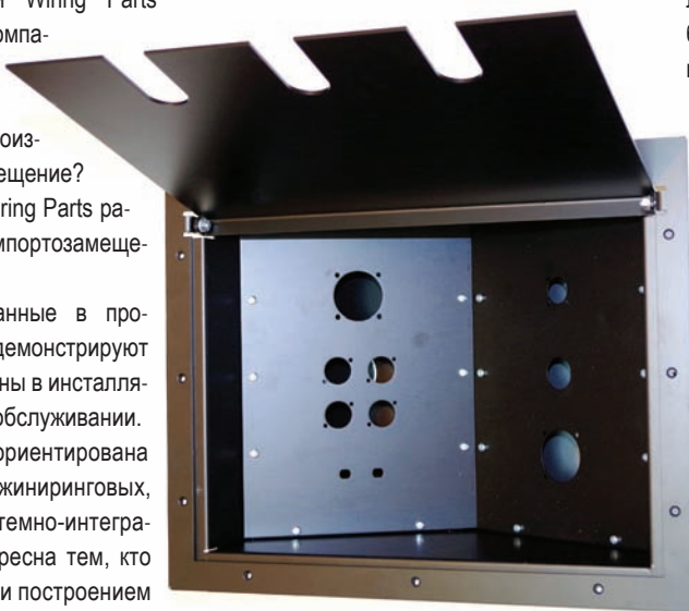
Люк сценический врезной в комплекте с монтажными панелями Wiring Parts WP-FPL
