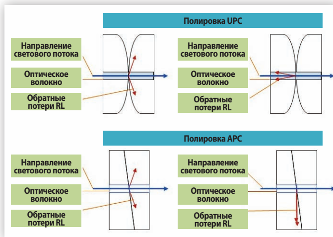
Способы полировки контактов оптических разъемов
